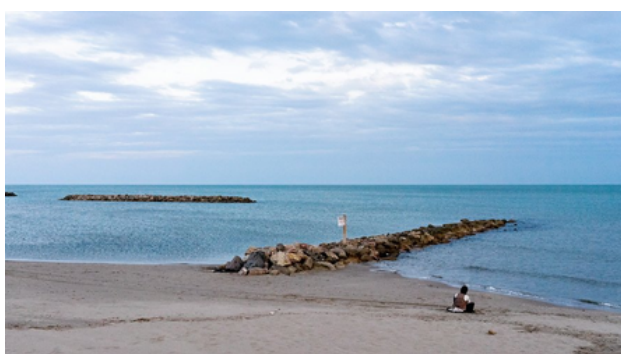
Transformation de l'épi en brise-lames à Vias (34)
